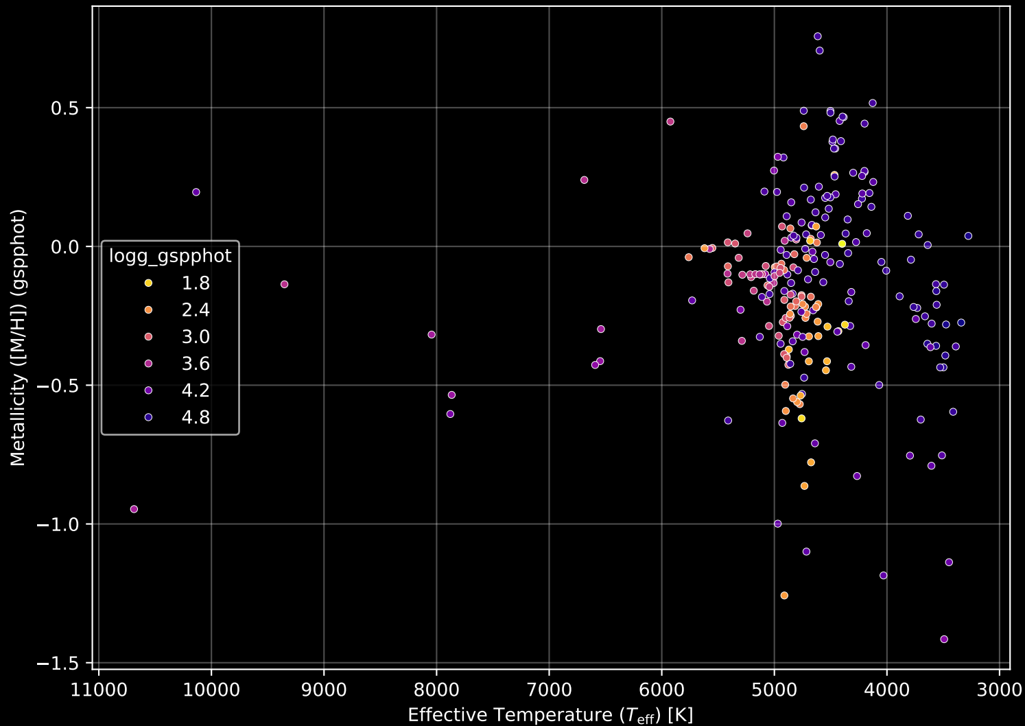
APOGEE DR17 Field: [120-24_btx] Stellar Population Parameters (n= 243)
